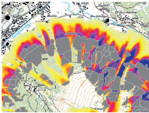
Abb 4 Szenario ohne Wald (grau: Lawinanrissgebiete, gelb-blau: Drücke der Lawinmodellierung analog zu Abbildung 2). Rreproduziert mit Bewilligung von Swisstopo (BA 081489).
