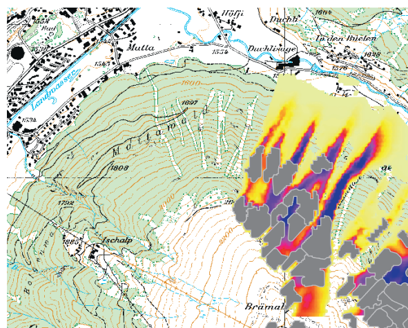
Abb 3 Klima- und Landnutzungsszenario, charakterisiert durch eine Erhöhung der Waldgrenze und Verdichtung der Waldstrukturen (grau: Lawinanrissgebiete, gelb-blau: Drücke der Lawinenmodellierung analog zu Abbildung 2). Reproduziert mit Bewilligung von Swisstopo (BA 081489).
